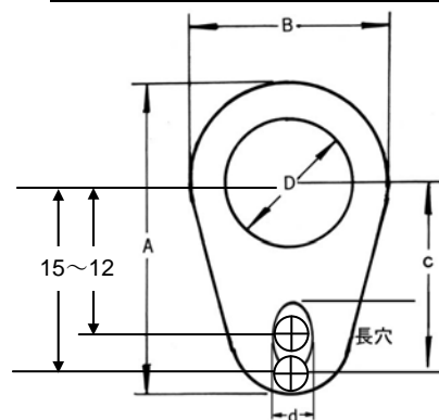
② 特殊フランジ 板厚 2.0mm
